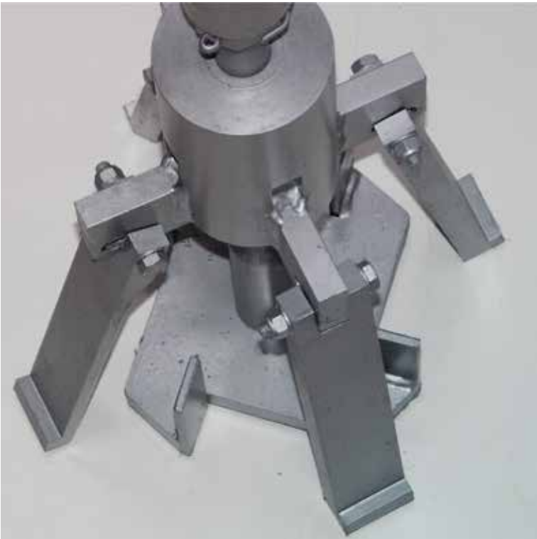
Abb. 2: Tiegelhebergerät Das Tiegelhebergerät wird für den Transport und Einbau des Tiegels eingesetzt.
